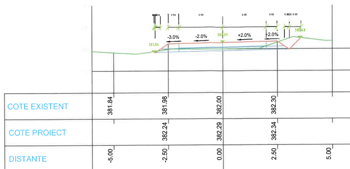
KM 390.00 Pichet nr.21
