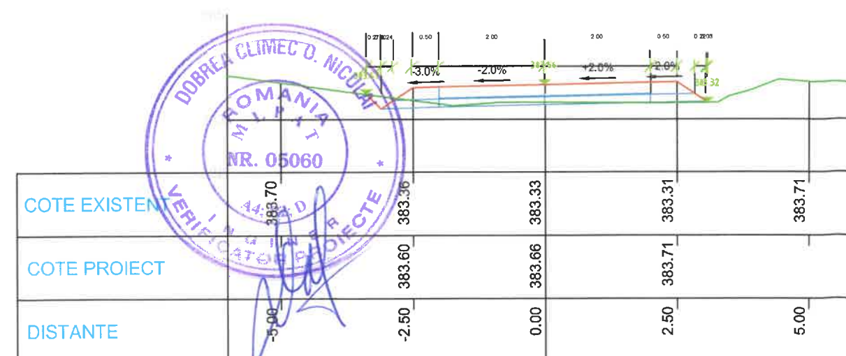
KM 450.00 Pichet nr.24
