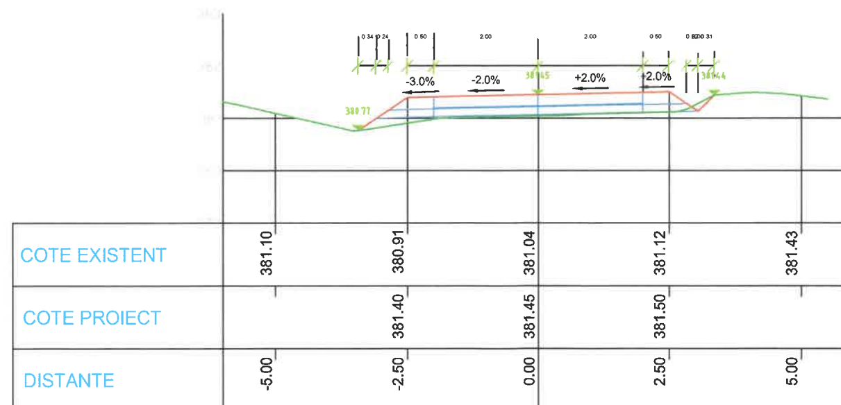
KM 360.00 Pichet nr.19
