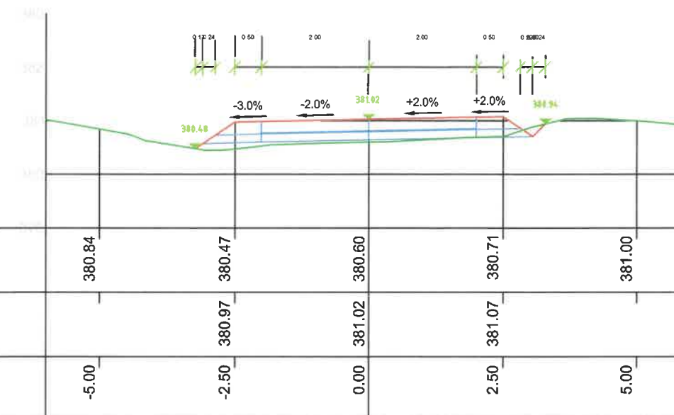
KM 346.14 Pichet nr.18
