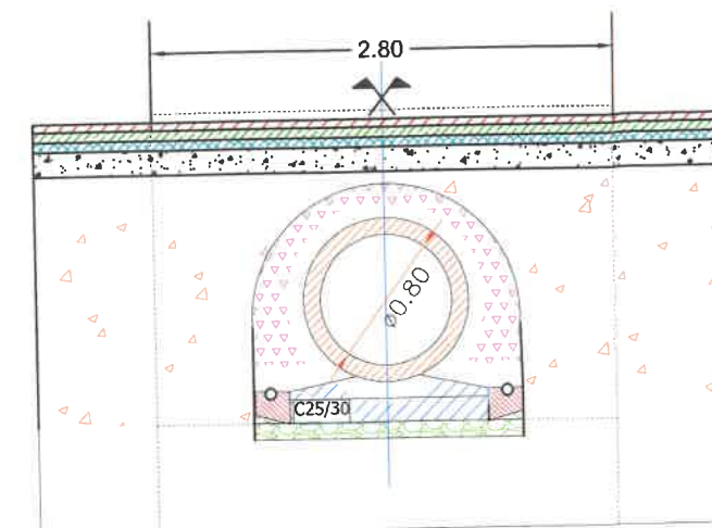
SECTIUNE D - D
